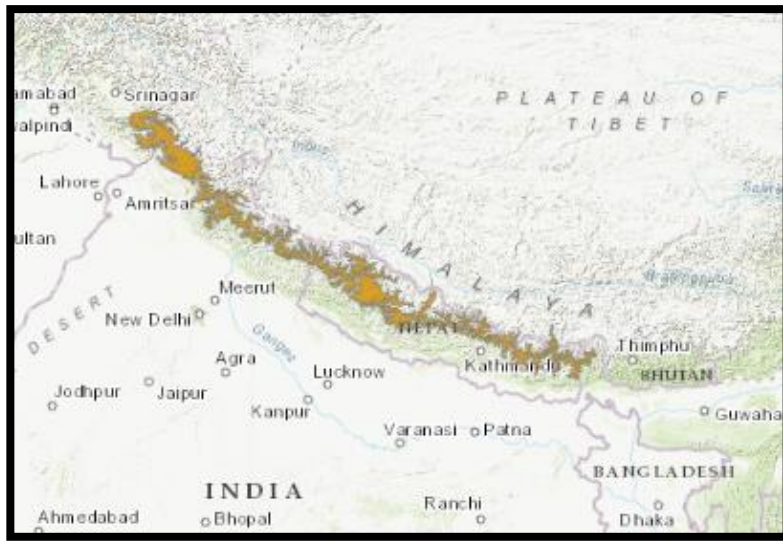
Aire de répartition du Hemitraqus jemlahicus , UICN
